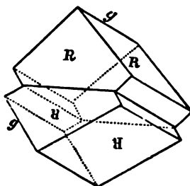
Calcite.
